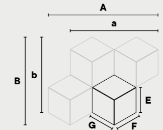
A 44,2 cm / 18" B 35,6 cm / 14" a 35,2 cm / 14" b 30,5 cm / 12" E 10 cm / 4" F 8,66 cm / 4" G 10 cm / 4"
